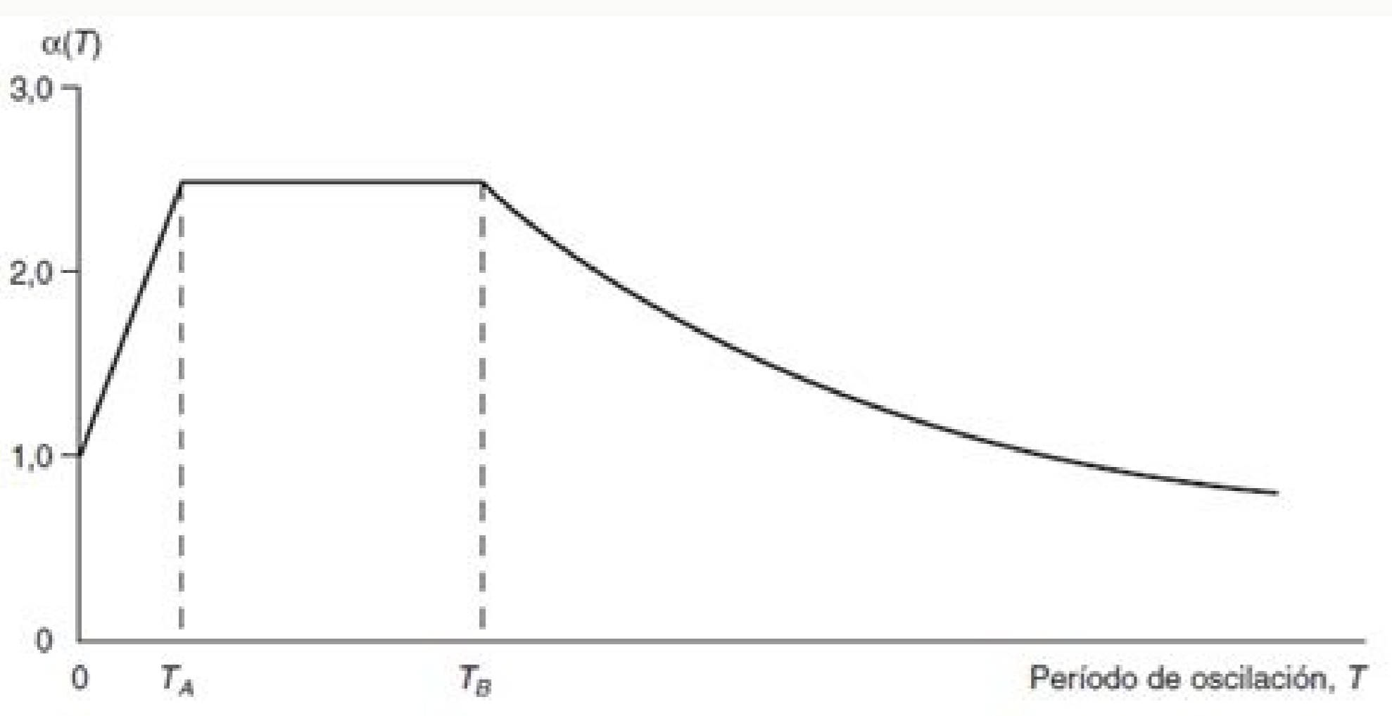
Figura 2.2. Espectro de respuesta elástica
